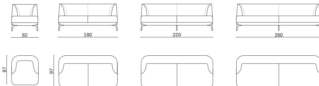
Elementi fissi poltrona e divani Armchair and sofa fixed units
